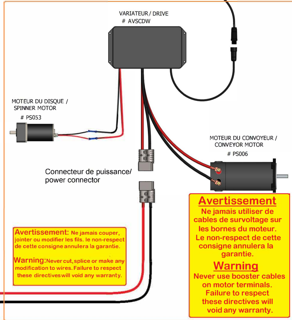
ARRIÈRE DE L'ÉPANDÉUR / REAR OF THE SPREADER
